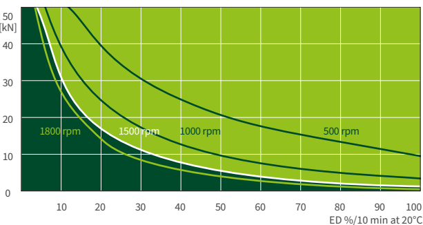
Ratio „N“ (7:1)
